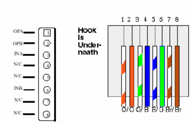
Ethernet connector (LAN)
